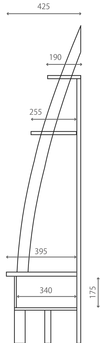
側面断面図
