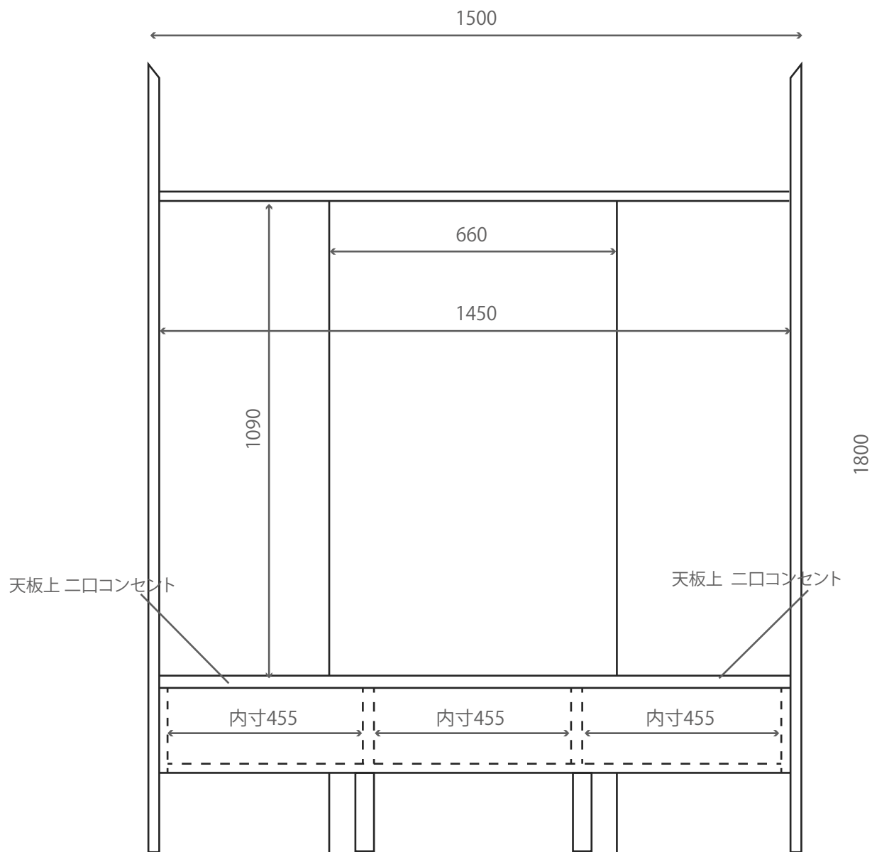
正面断面図
