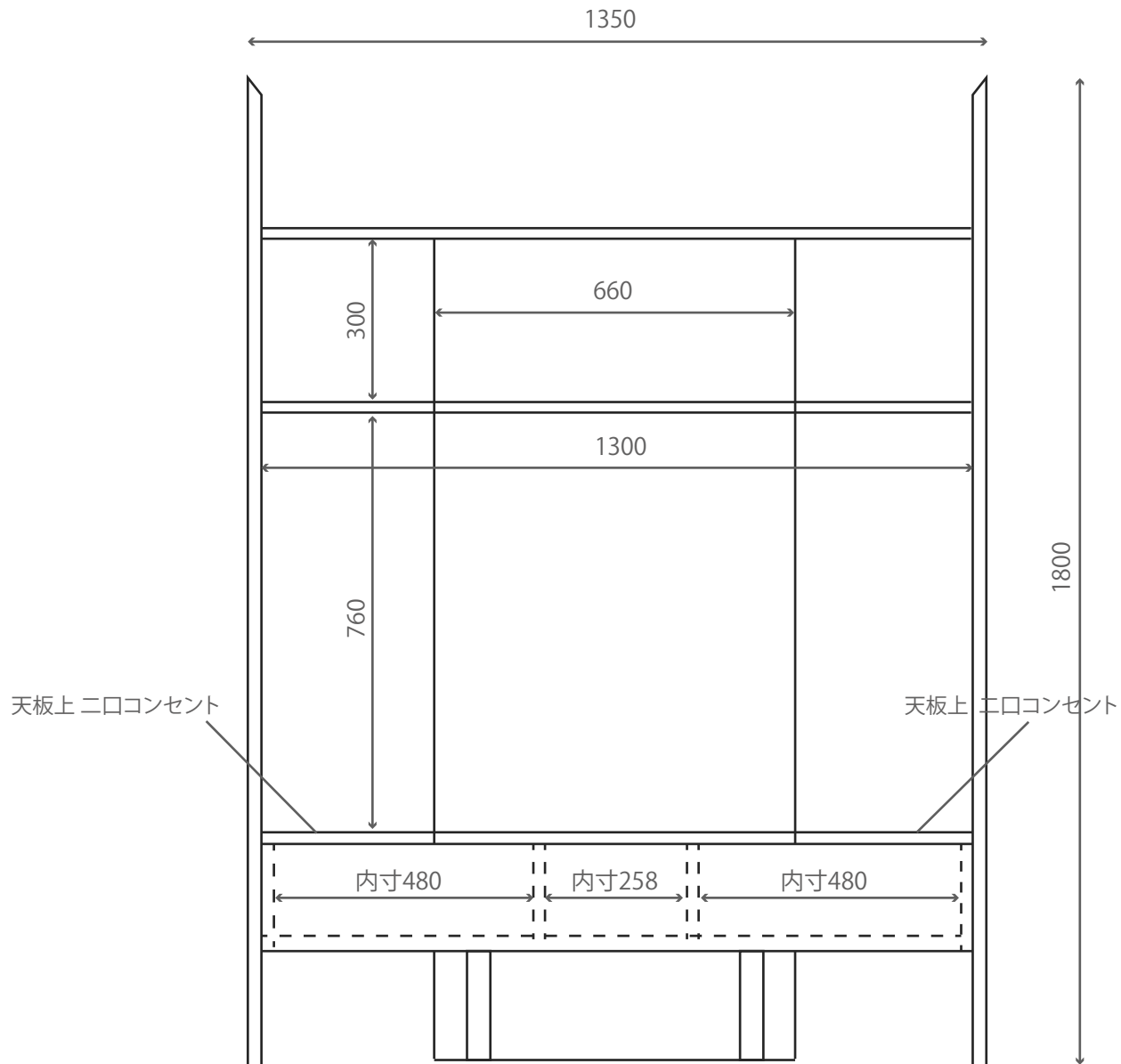
正面断面図
