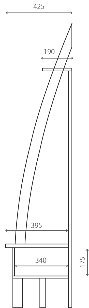
側面断面図
