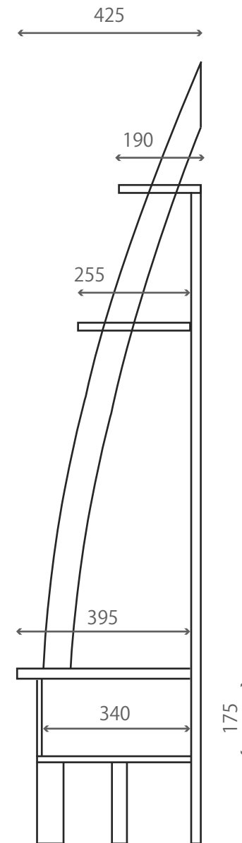
側面断面図
