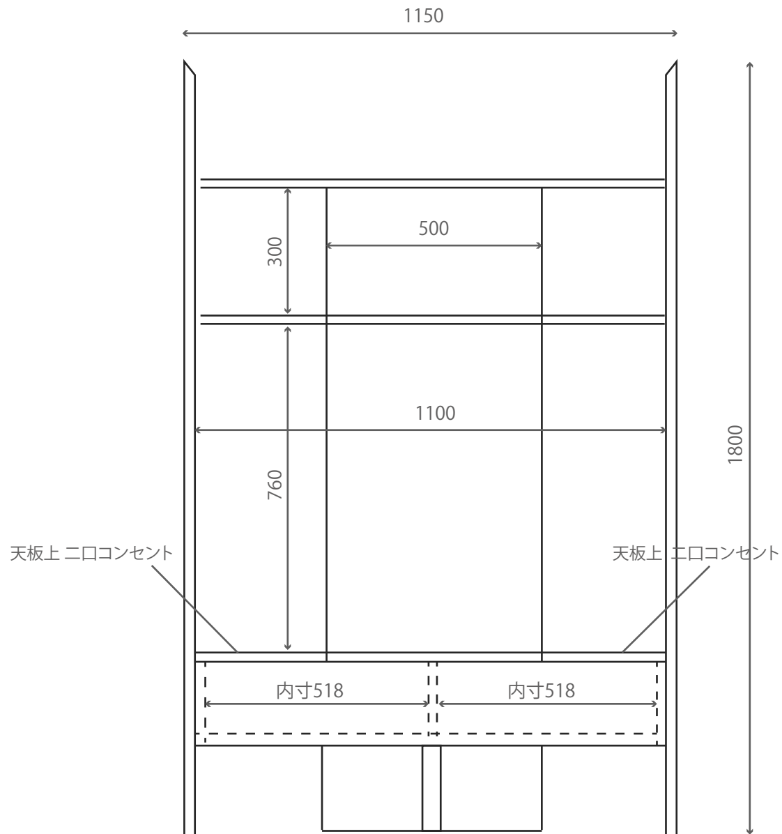
正面断面図
