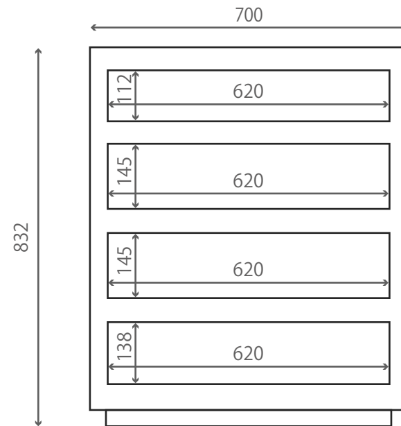
幅700mm キャビネット
